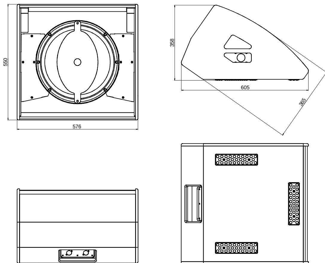
Рис.3. Габаритные размеры
