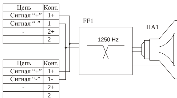
Рис.2. Схема электрическая структурная
