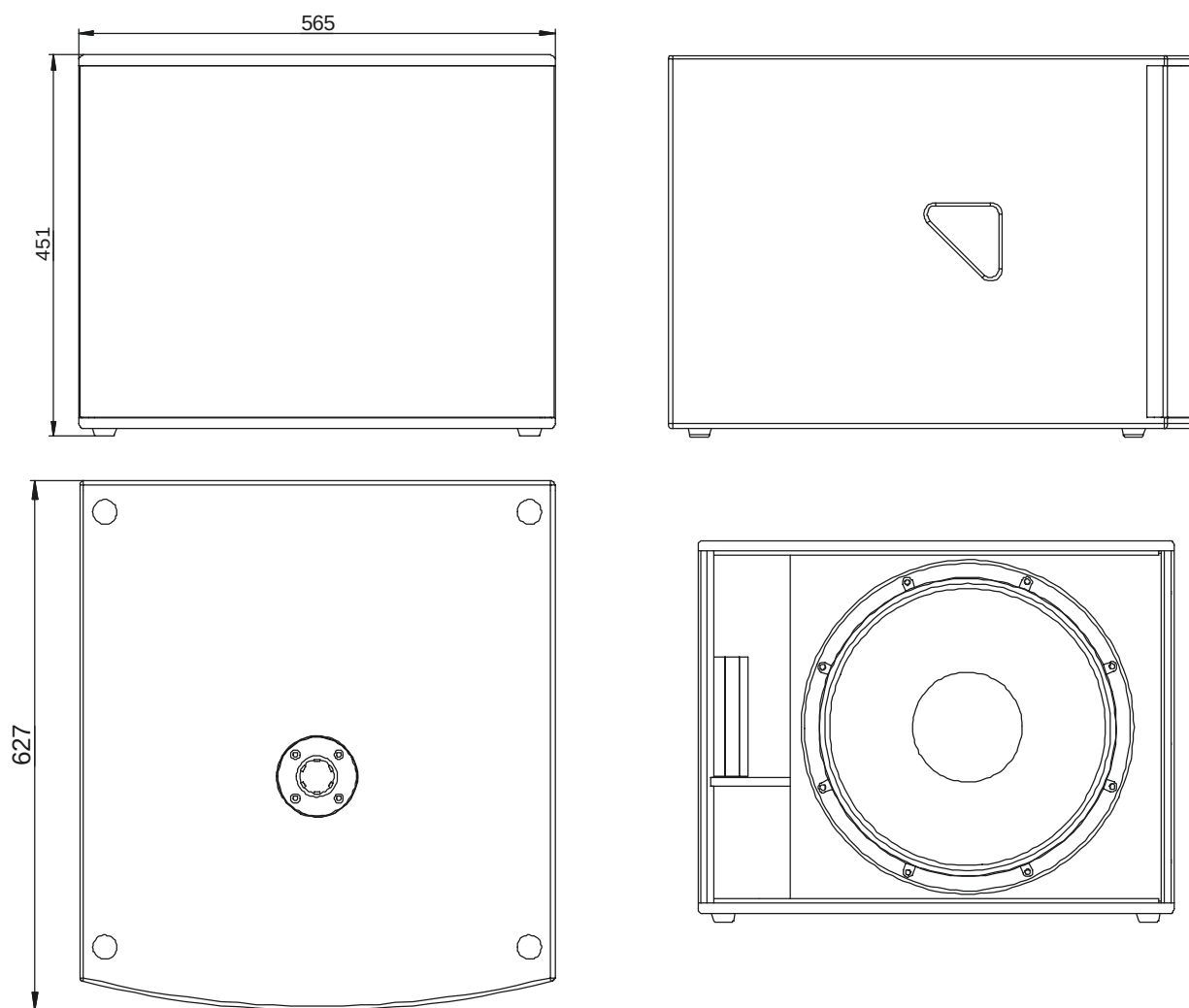
Рис.3. Габаритные и присоединительные размеры
