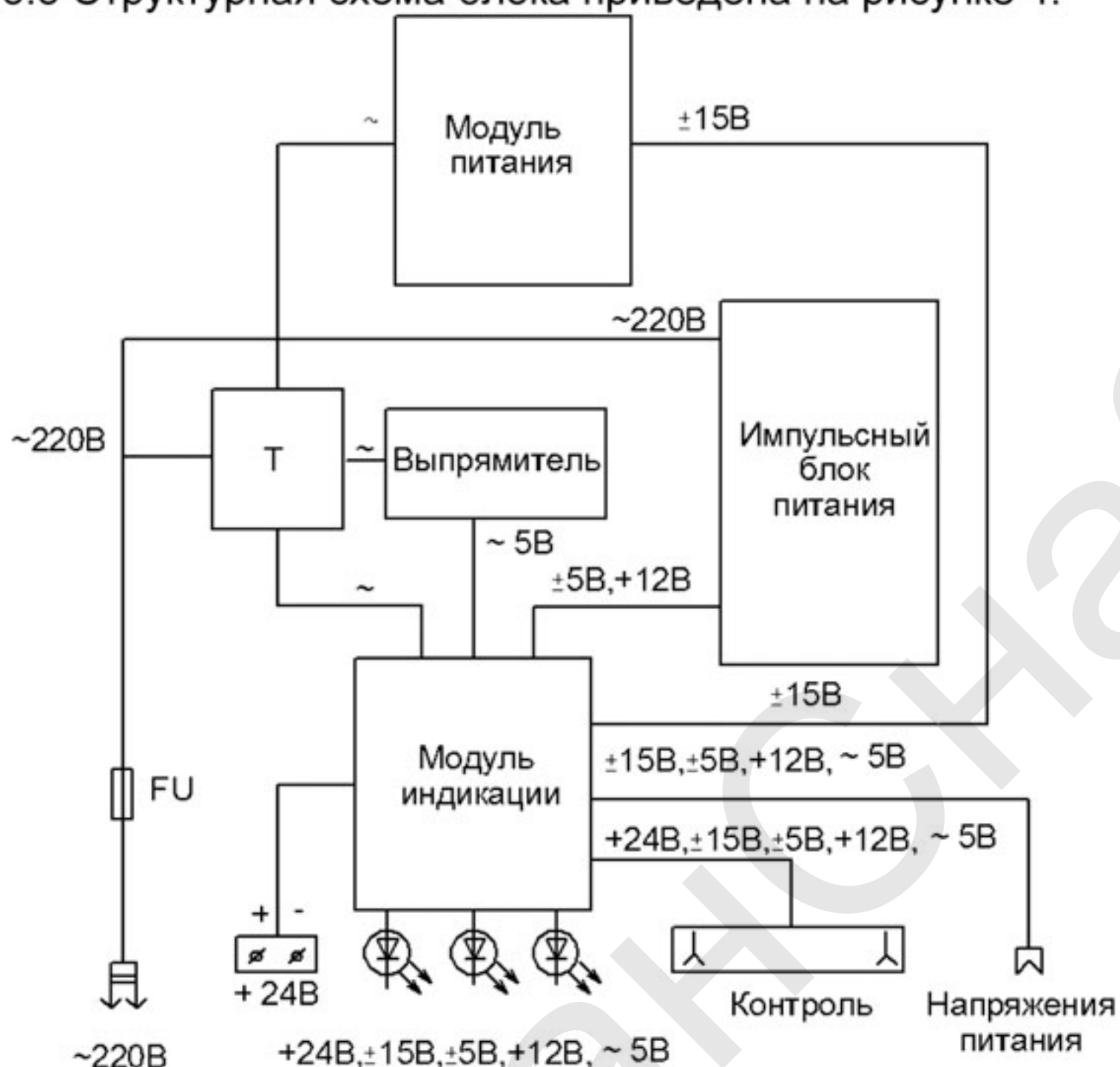
Рисунок 4 – Блок питания стабилизирующий БПС-7. Схема структурная.
