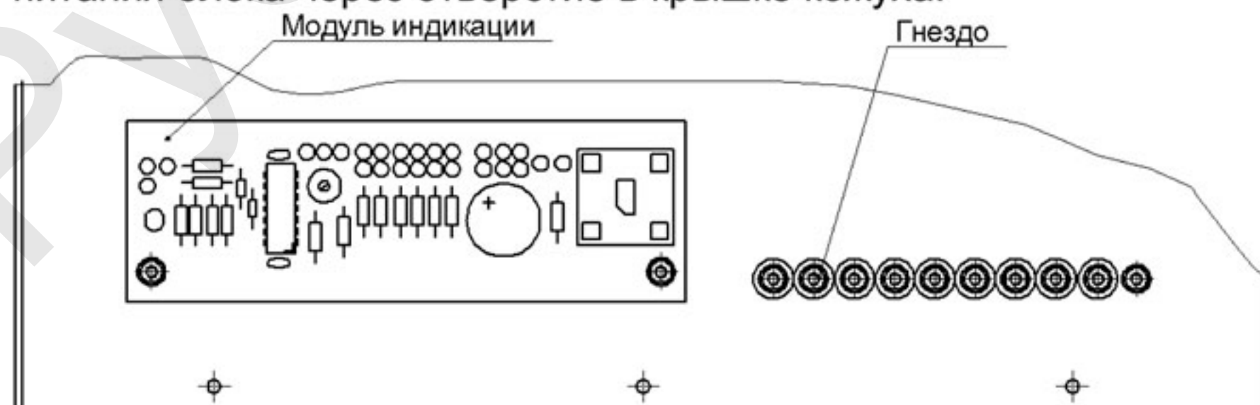
Рисунок 3 – Модуль индикации. Внешний вид.
