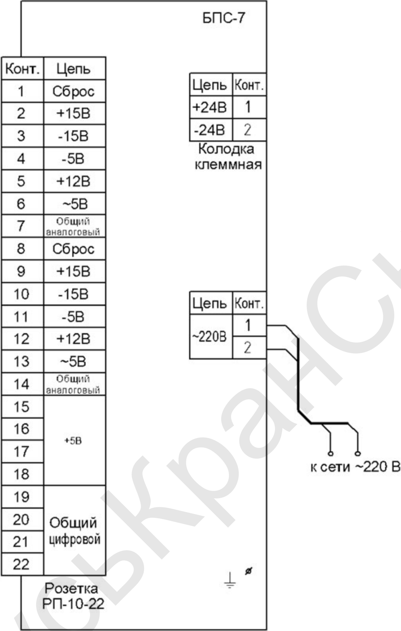
Рисунок 5 – Блок питания стабилизирующий БПС-7. Схема подключения.
