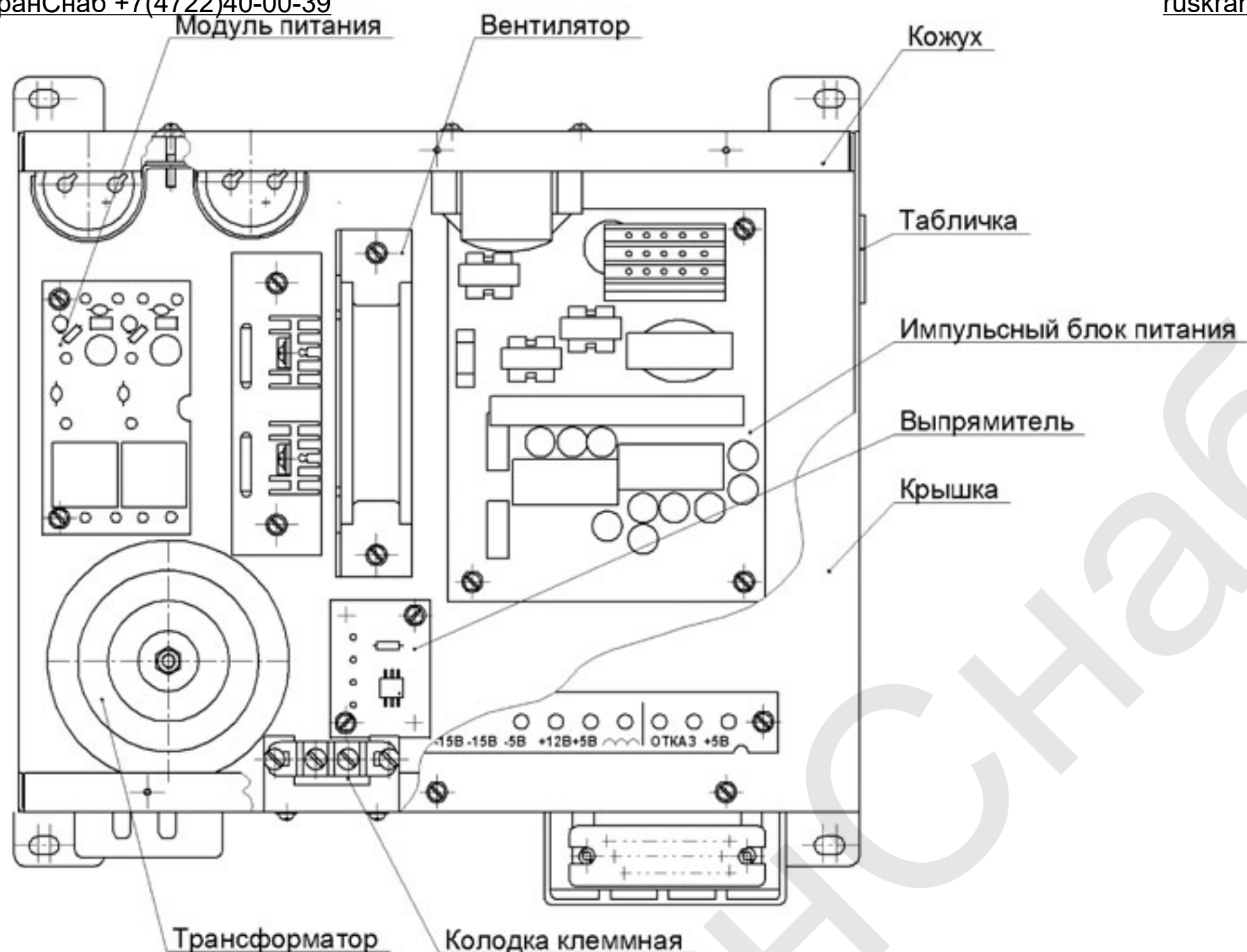
Рисунок 2 – Блок питания стабилизирующий БПС-7. Вид внутри.
