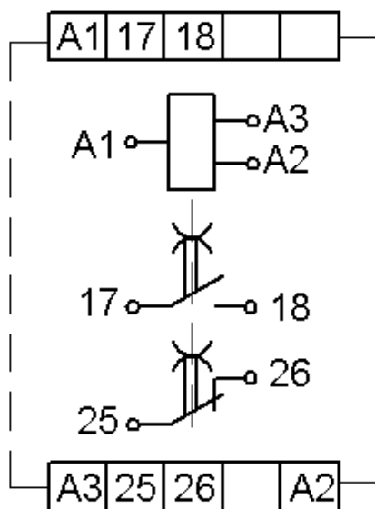
Рисунок 2 - Схемы подключения реле
