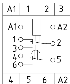
ВЛ73А
