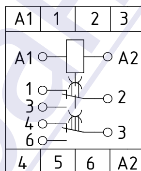
ВЛ78А
