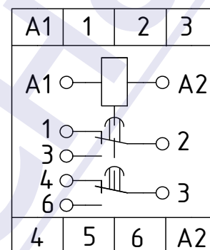
ВЛ76А
