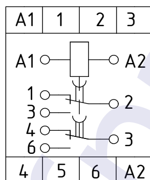
ВЛ77А, ВЛ79А
