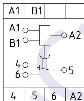
ВЛ74А, ВЛ75А
