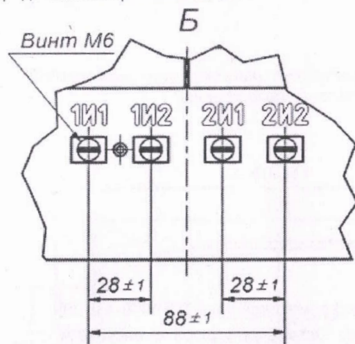
Рисунок А.6 – Габаритный чертеж. Расположение контактов вторичных обмоток трансформаторов тока ТПЛУ-10-1.2.
