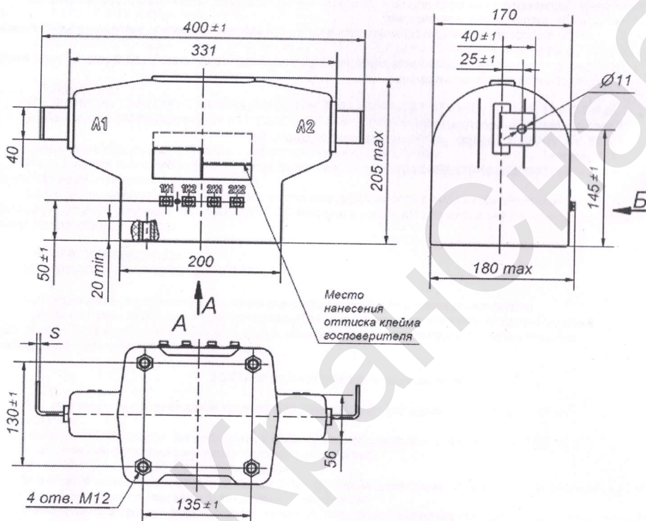
Рисунок А.1 – Габаритный чертеж трансформатора тока ТПЛУ-10-1.2-1В для номинальных первичных токов от 10 до 100 А включительно. Остальное смотри в таблицах А.1 – А.2.
