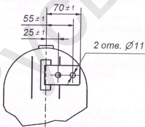
Рисунок А.2– Габаритный чертеж выводов первичной цепи трансформаторов тока ТПЛУ-10-1.2-2В для номинальных первичных токов от 10 до 600 А включительно. Остальное смотри на рисунке А.1.
