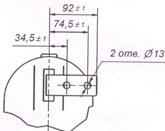
Рисунок А.3 – Габаритный чертеж выводов первичной цепи трансформаторов тока ТПЛУ-10-1.2-2В для номинальных первичных токов от 10 до 1000 А включительно. Остальное смотри на рисунке А.1.
