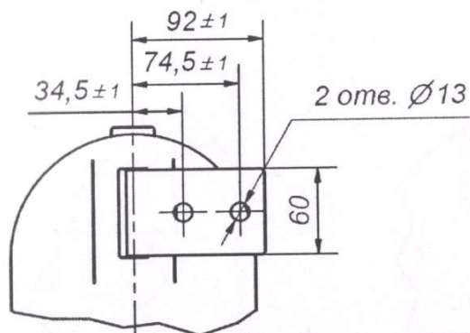
Рисунок А.4 - Габаритный чертеж выводов первичной цепи трансформаторов тока ТПЛУ-10-1.2-2В для номинальных первичных токов от 10 до 1500 А включительно. Остальное смотри на рисунке А.1.
