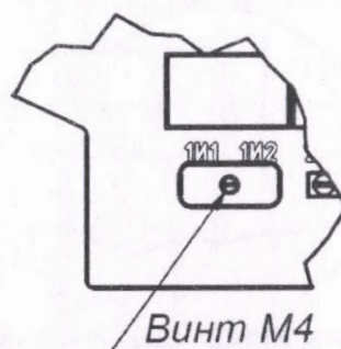
Рисунок А.7 – Габаритный чертеж. Защитная крышка для пломбирования вторичных выводов трансформаторов тока ТПЛУ-10-1.2.
