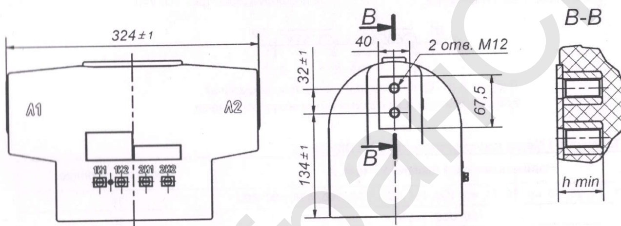
Рисунок А.5 – Габаритный чертеж трансформаторов тока ТПЛУ-10-1.2-Т для номинальных первичных токов от 10 до 1000 А включительно. Остальное смотри на рисунке А.1 и в таблице А.3.
