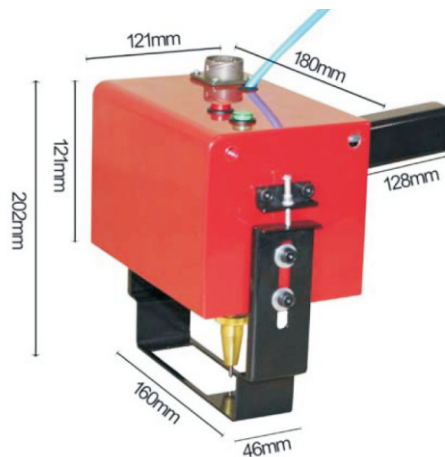
Портативная голова 75x25мм (размеры)
