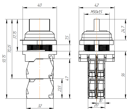
Рис.2. Переключатель управления с рукояткой.
