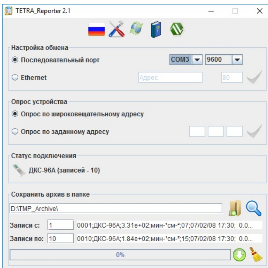
Рисунок 6 Рабочее окно программы TETRA_Reporter 2.1
