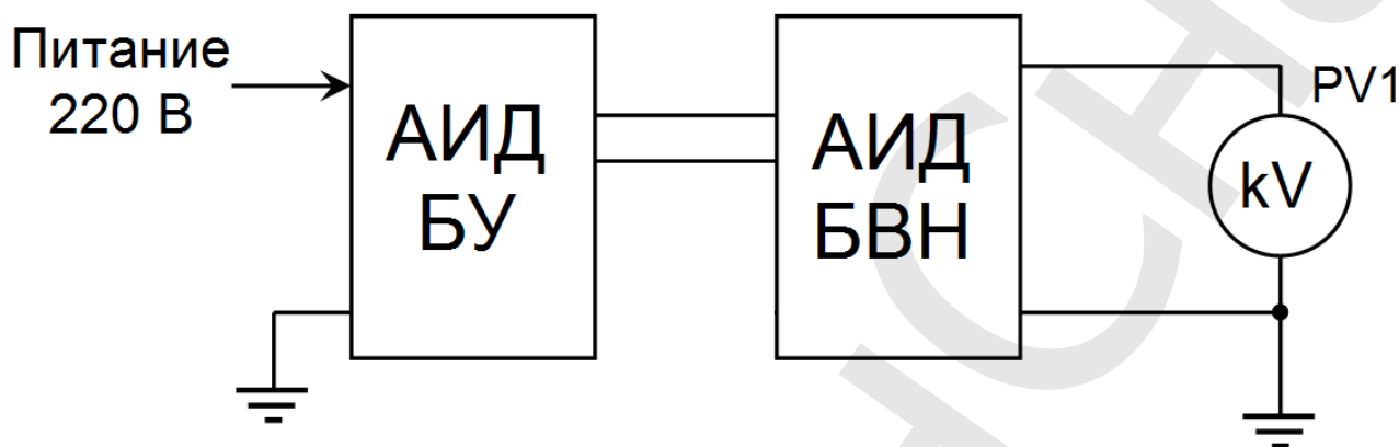
Рисунок 9 – Схема соединений при определении погрешности измерений переменного испытательного напряжения Аппарата
