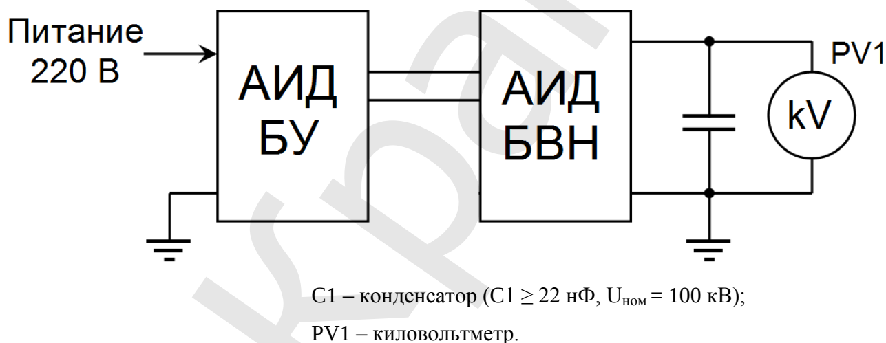
Рисунок 11 – Схема соединений при определении погрешности измерений выпрямленного испытательного напряжения Аппарата
