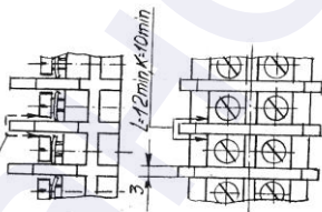
Рис. 10. Устройство и средства взрывозащиты ящика клемного с кабельными вводами CAPRY LCIE 84-6109xEelI(ex)
